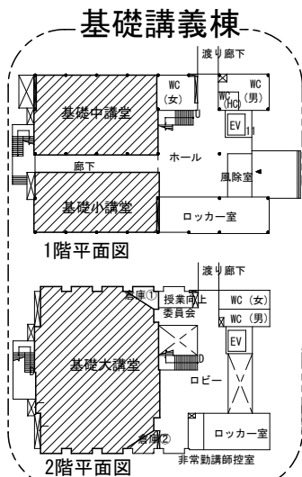
2階平面図
