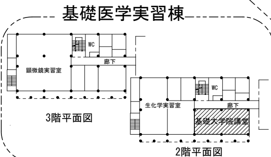
2階平面図
